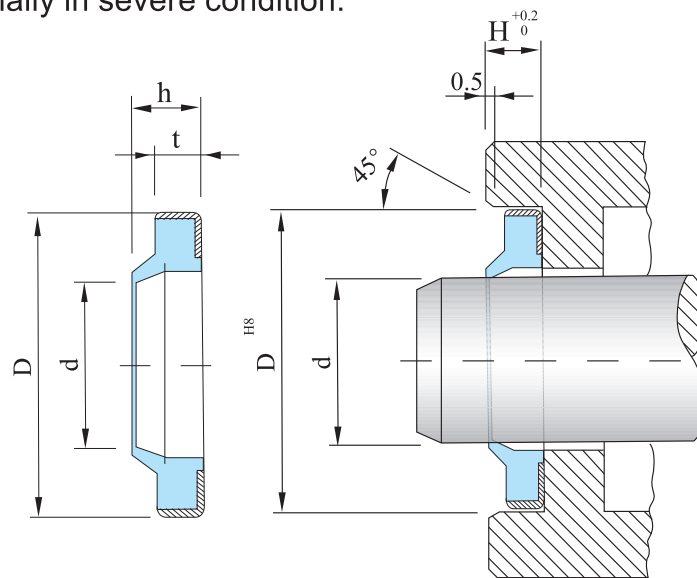
GA型式-油封規格表 GA Type Size List
