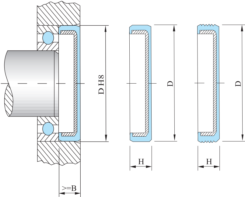
VK型油封規格表 VK Type End Cap Size List
