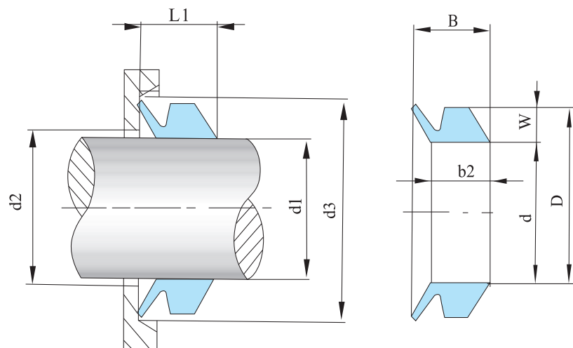
VS型油封規格表 VS Type Size List
