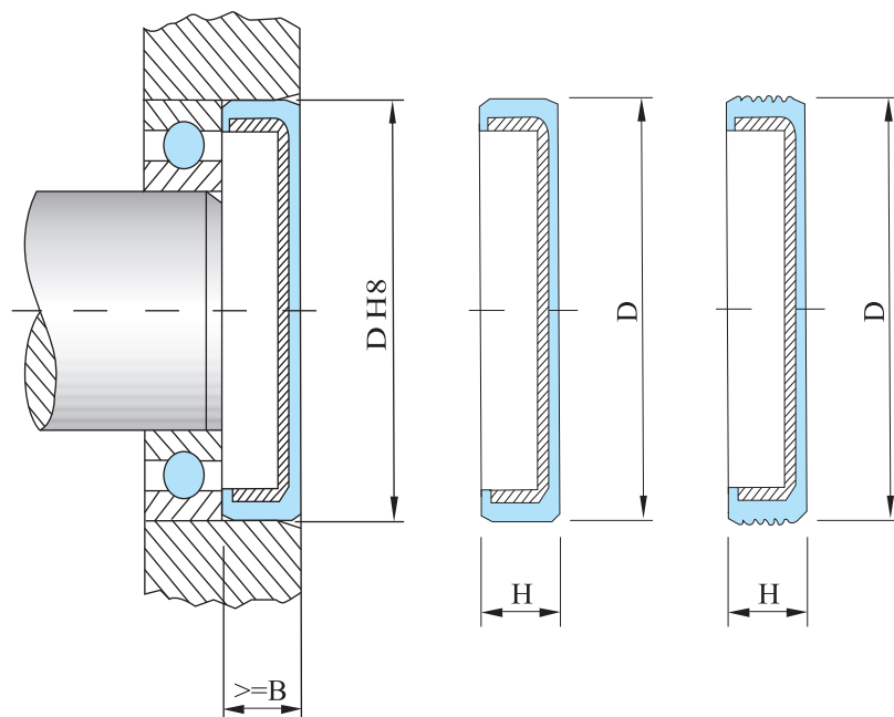
EC型油封規格表 EC Type End Cap Size List
