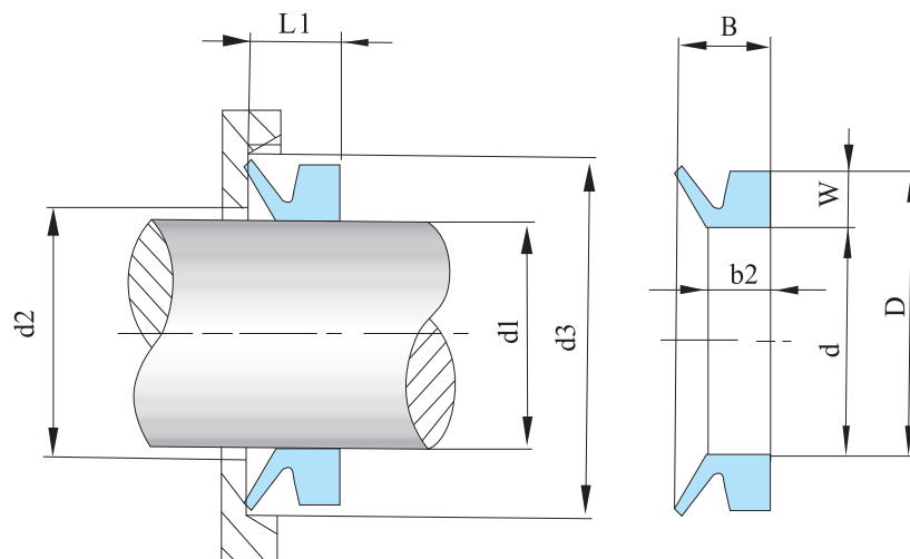
VA型油封規格表 VA Type Size List
