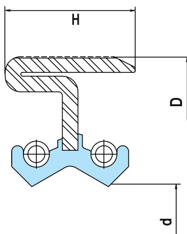
DB型油封规格表 DB Type Seal Size List
