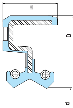
DC型油封规格表 DC Type Seal Size List
